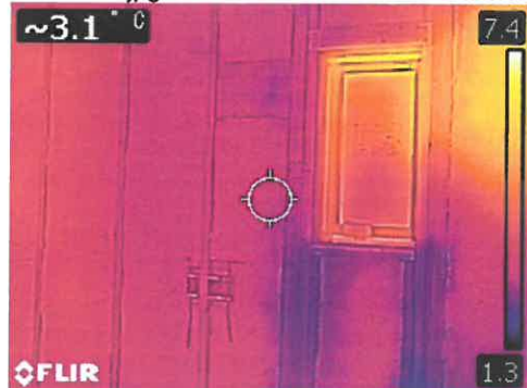
FLIR0549.jpg 2022/12/10 13:23:32
